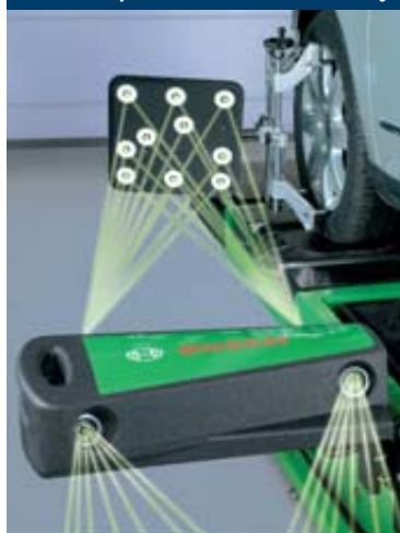
Merací senzor
